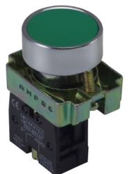
XB2-BA31 Material: Metálico Faceado Contato: 1 NA Cor: Verde
