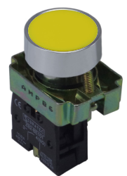
XB2-BA51 Material: Metálico Faceado Contato: 1 NA Cor: Amarelo
